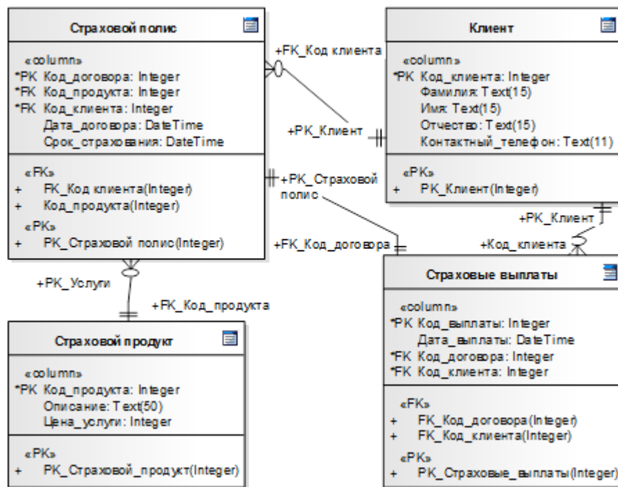
Рисунок 2 – Модель базы данных АИС страхования
