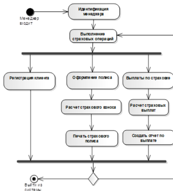
Рисунок 3 – Диаграмма деятельности
