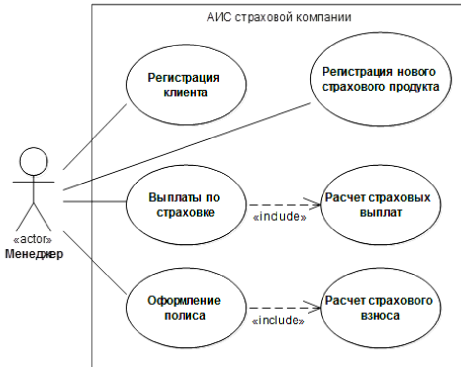
Рисунок 1 – Модель вариантов использования
